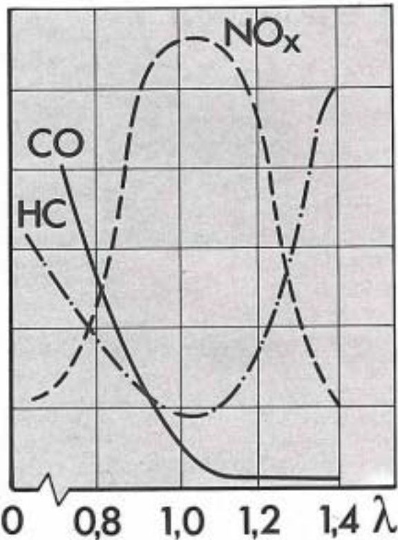
Schadstoffkennlinien beim Ottomotor
