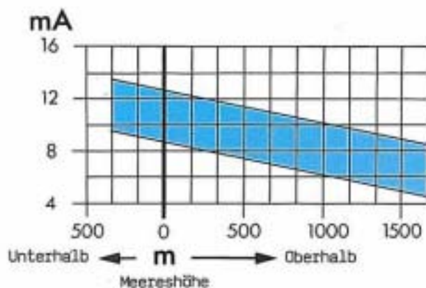
Verstellbereich des Höhenbarometers
